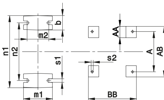
Flange
